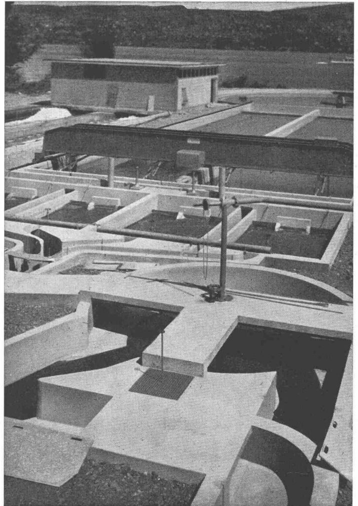
Kläranlage Horgen/Zürichsee
