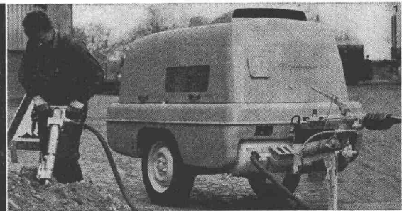
neuer, lärmärmer, vollkommen luftgekühlter 4 m³-Kompressor
