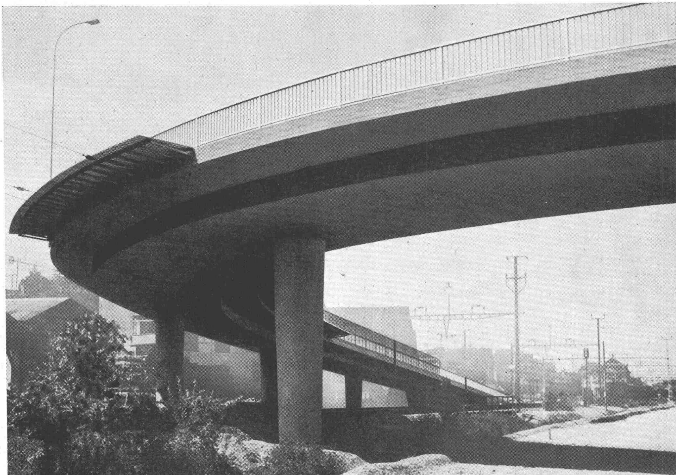
Zollbrücke Rheineck, mit Barralent betonierte
