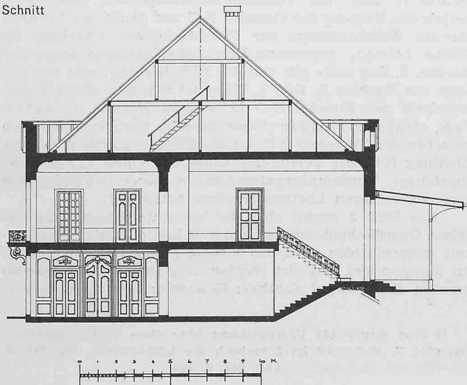
Schnitt
