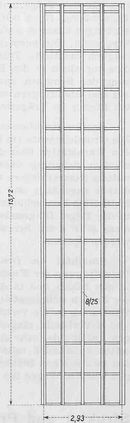
Bild 16 (rechts). Ansicht des Rostelements, Masstab 1:150
