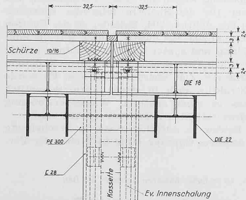
Bild 11 (oben). Anschluss der Kassette an die Schürze, Horizontalschnitt 1:20
