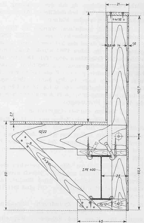
Bild 9. Brüstung, Masstab 1:20
