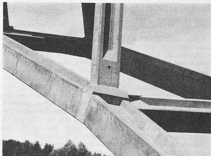
Bild 9. Knotendetail über dem Stabbogen. Man erkennt den Ortsbeton des Fugenschlusses an seiner helleren Farbe
