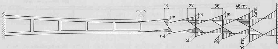
Bild 3. Ueberhöhtes Längsprofil der ausgeführten Brücke; Längenmasstab 1:2000, Höhenmasstab 1:800
