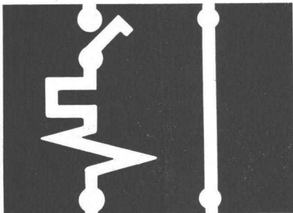
SL mit trennbarem Nulleiter
