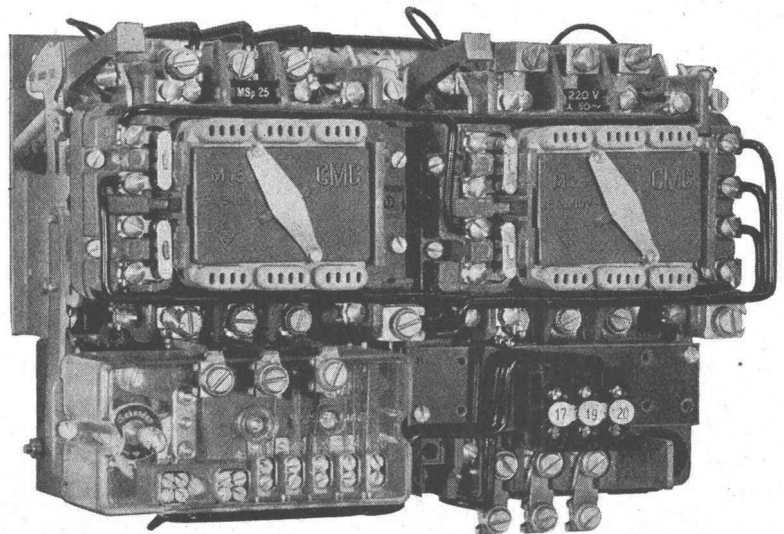
Sterndreieckschütz Typ MSp 15/25
