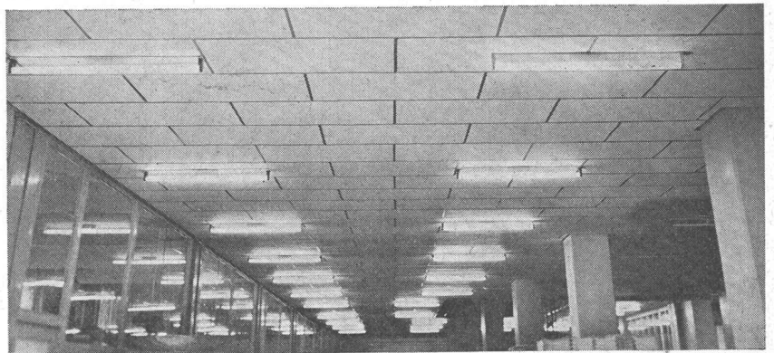
ungelochte Schallschluckplatte, unbrennbar, hier mit sichtbarem Hängeros in einem Druckereisaal
