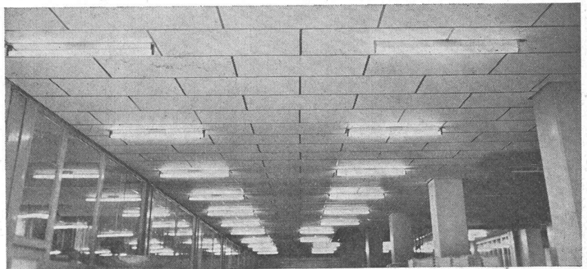
ungelochte Schallschluckplatte, unbrennbar, hier mit sichtbarem Hängeroast in einem Druckereisaa
