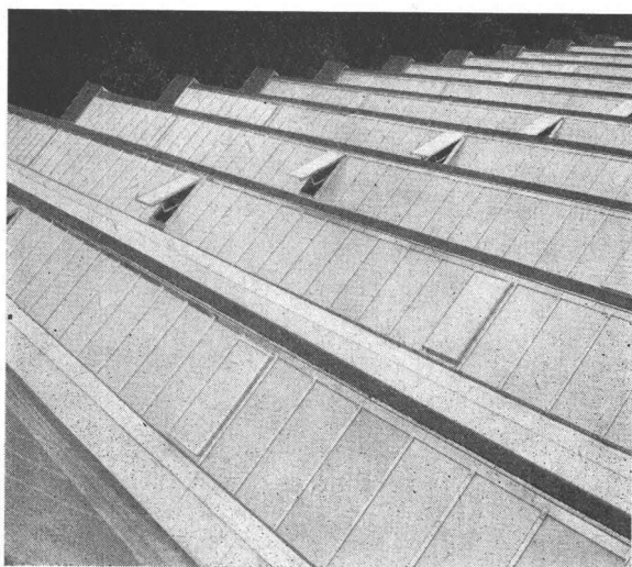
Shed-Fenster in kittloser Konstruktion System WEMA
