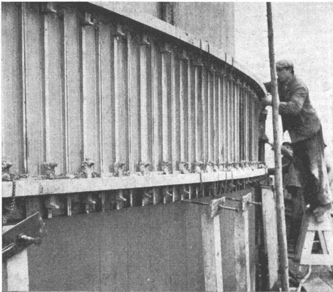
Schalung im Hochbau
