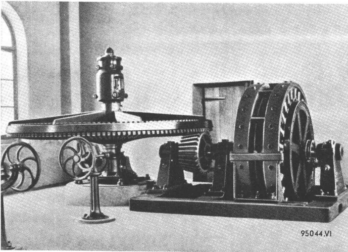
▲ Elektrizitätswerk Kappelerhof Baden. 175-kVA-Generator
