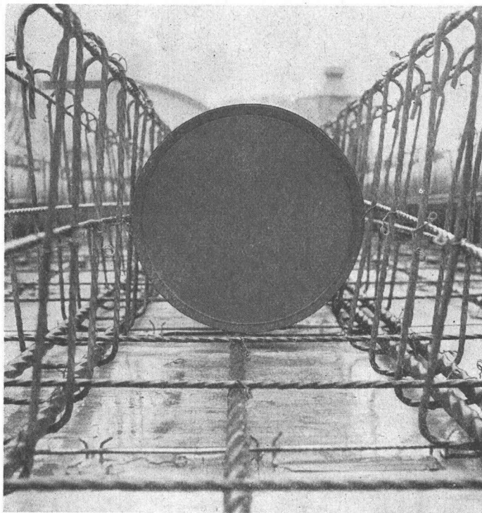
Ausparungs- und Schalungsrohre aus Hartpapier für Betonbauten. \varnothing bis 565 m/m. Längen nach Wunsch.
