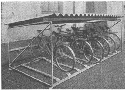
Serien-Fahrradklammern mit Ueberdachung und Einfahrkufen für hoch-tief-gestellte Fahrräder. Typ KU 10
