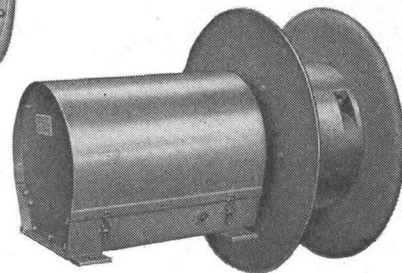
Federkabeltrommel Typ AFM
