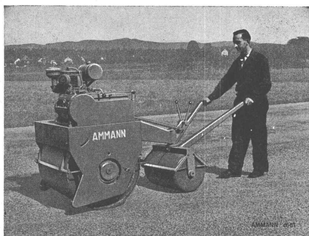
Selbstfahrende Vibrowalze Type LM, mit Lenkwalze
