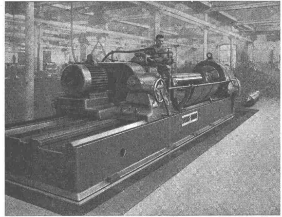
Isolierte Walzenschleifmaschine
