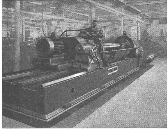
Isolierte Walzenschleifmaschine
