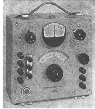
Volltransistor. Präzisions-Messbrücke
