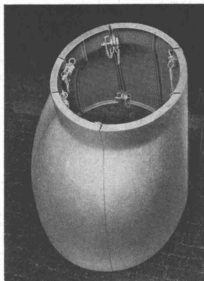
Exzentrische Kuppel- Schalungen für Vertikal- schächte
