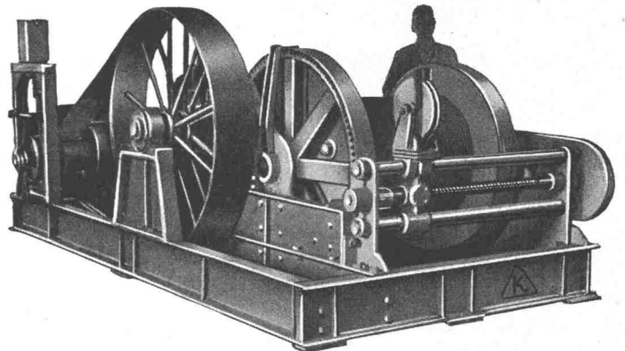
Type KS 50/80 mit 2 Geschwindigkeiten Zugkraft 5000 kg, mit elektr. Ausrüstung
