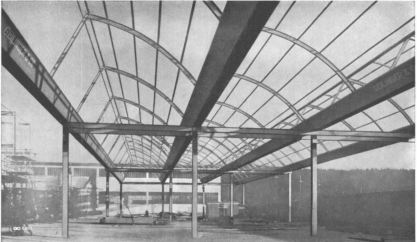
Shedkonstruktion mit rinnenförmigen Hauptträgern (+ Pat. angem.)
