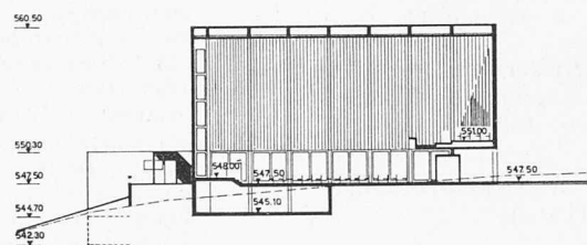
Längsschnitt Kirche
