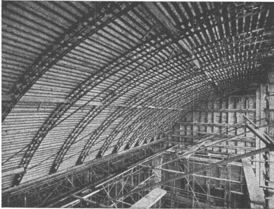
Shed-Dach mit Schalungsträger und BK
