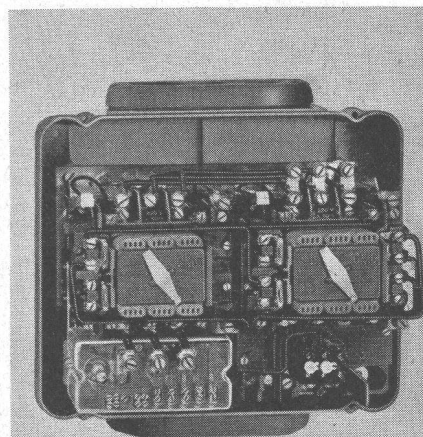
Sterndreieckschütz CMSp 25
