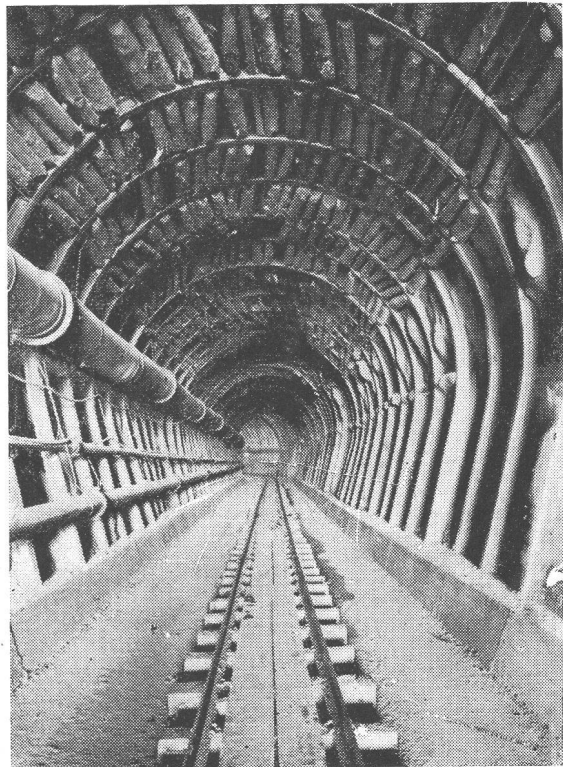
Stollen mit Stahleinbau in gebrächem Fels
