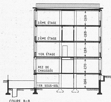
COUPE B-B
