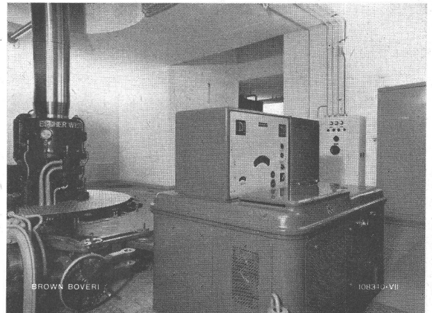
Bild 2. Elektrischer Turbinenregler in der Zentrale Fionnay (Mauvoisin). Rechts der Apparatekasten mit den verschiedenen elektrischen Kreisen, in der Mitte das Steuerwerk und links das Wellenende und der Leitapparat der Turbine
