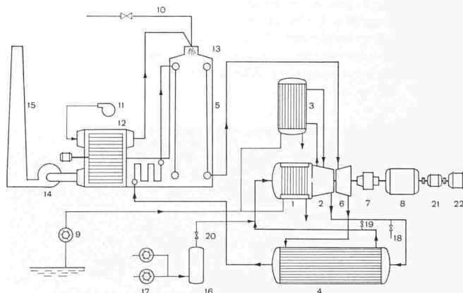
Bild 2. Schema der Anlage Toyotomi
