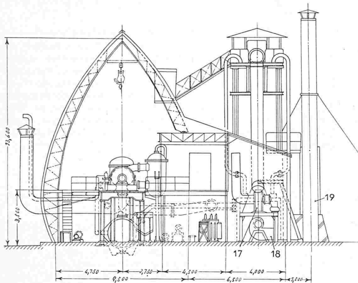
Bild 6. Dispositionsplan der Anlage Toyotomi 1:250
