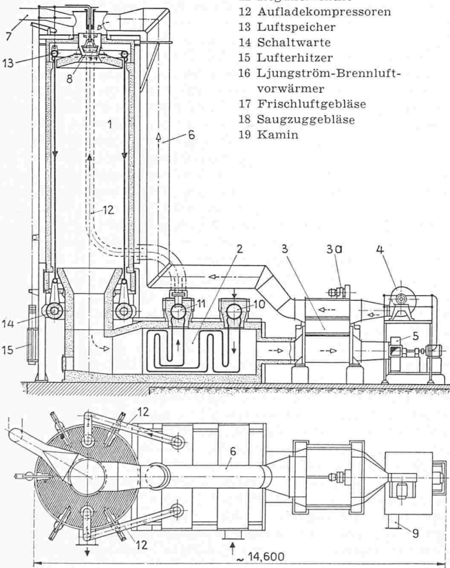
Bild 5. Lufterhitzer, rd. 1:180
