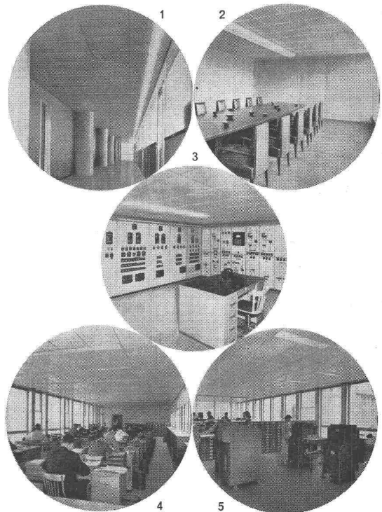
1. Korridor: ZENT-FRENGER-Deckenheizung mit Schallschluck 2. Sitzungszimmer: ZENT-FRENGER, Lüftung u. Schallschluck 3. Schaltraum: Zuleitungen hinter der ZENT-FRENGER-Heizungsdecke. 4. Bureau: Angenehmes Klima dank ZENT-FRENGER-Strahlungsheizung, Lüftung und Schallschluck 5. Lochkartenraum: ZENT-FRENGER-Heizung mit Schallschluck
