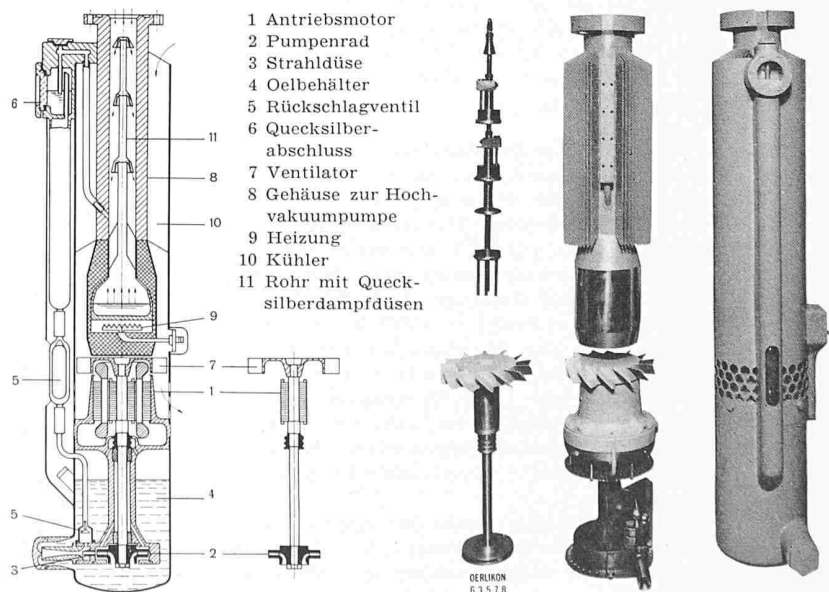
Bild 1. Die Oerlikon-Hochvakuum-Strahlpumpe
