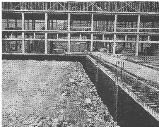
Trennwandisolation im Shed des Einsiedler Neubaus der Firma Landis & Gyr AG. mit AFRATAR
