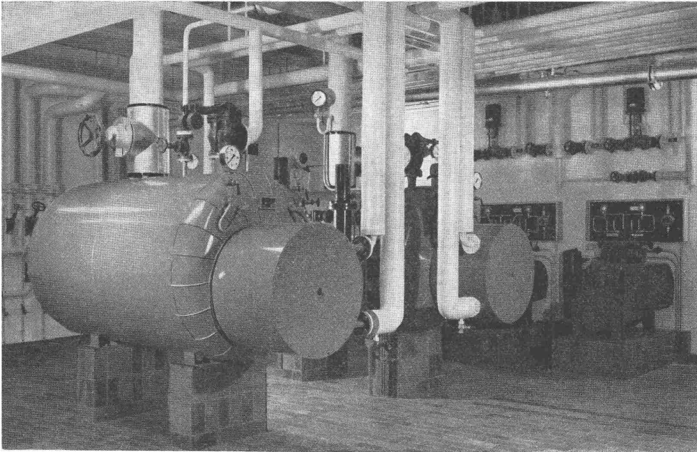
Heißwasser-Dampfumformer
