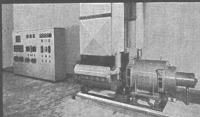
100 kW Notstromanlage
