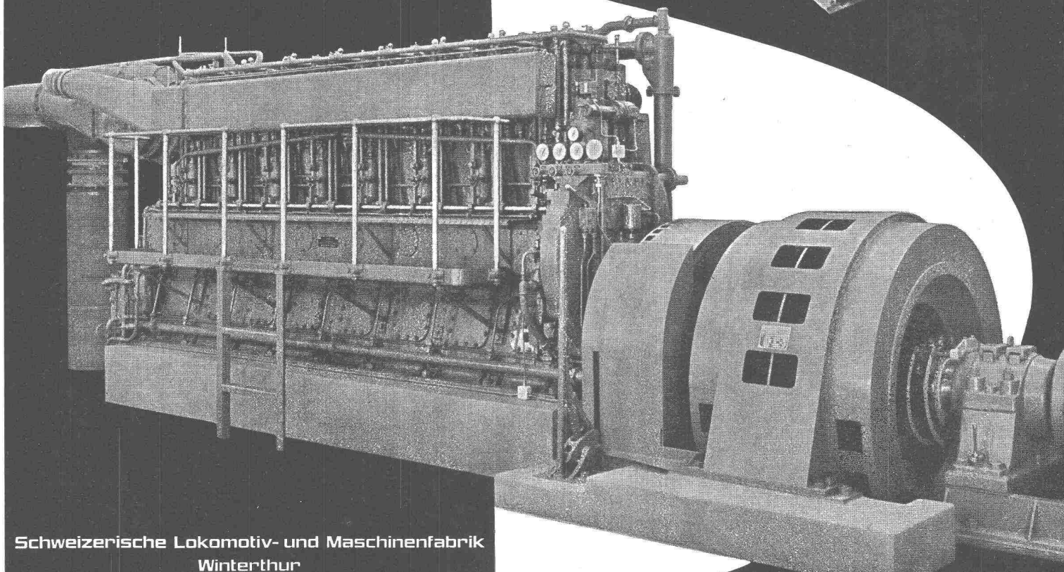
750 kW Notstromgruppe
