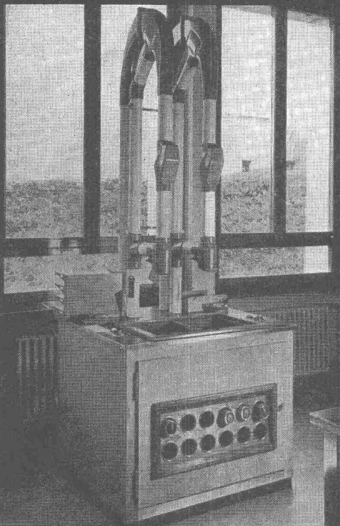
Zentralstelle einer Anlage mit 2 Rohrkreisen und druckknopfgesteuerten Weichen
