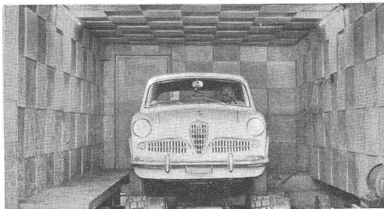
Versuchswagen auf dem Rollprüfstand für akustische Messungen
