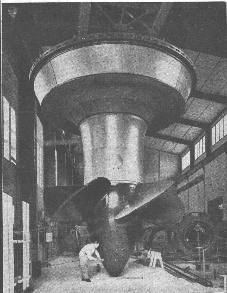
LAUFRAD 5 m Ø
