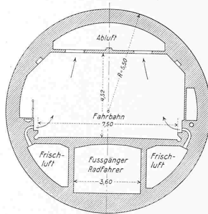
Tunnelquerschnitt 1 : 200
