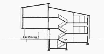
Haupttrakt
