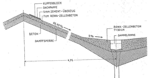
Maschinenhaus der Kraftwerk AG., Birsfelden 4000 m 2 ROWA ZB 9, 120 m 3 für Rinnen, Raumgewicht: 550 kg/m 3 . Bauleitung: Ingenieurbüro A. Aegerter & Dr. O. Bosshardt AG., Basel.
