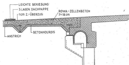
Fabrikgebäude der Firma Heberlein & Co., Wattwil SG 2500 m 2 ROWA ZB 8, Raumgewicht ca. 500 kg/m 3 . Bauleitung: Ingenieurbüro E. Frei & E. Krauer, Rapperswil SG.
