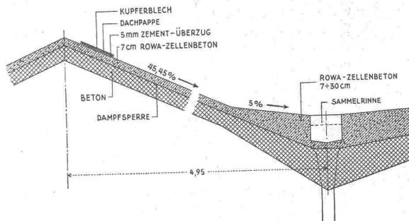
Maschinenhaus der Kraftwerk AG., Birsfelden 4000 m 2 ROWA ZB 9, 120 m 3 für Rinnen, Raumgewicht: 550 kg/m 3 . Bauleitung: Ingenieurbüro A. Aegerter & Dr. O. Bosshardt AG., Basel.
