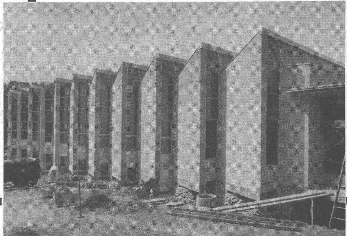
Ausfachung eines Beton-Skeletthaues
