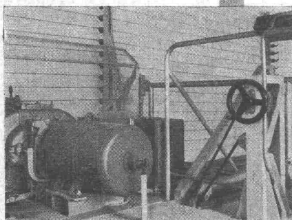
Elektronisch gesteuerte Flügel- prüfanlage für stufenlosen Regel- bereich von 1:900
