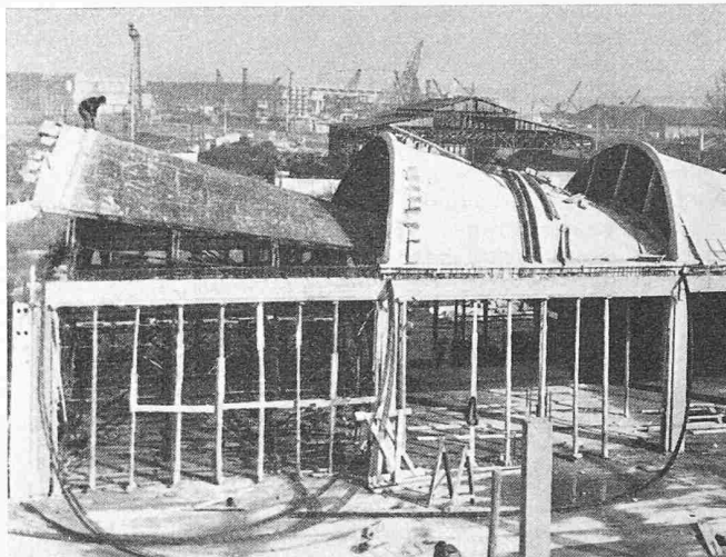
Bild 3. Oberflächenbehandlung von Betongewölben mit VC-Matten, Ausschulfrist 2 Tage (Bordeaux, Frankreich)
