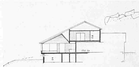
Schnitt Gaststube 1:600
