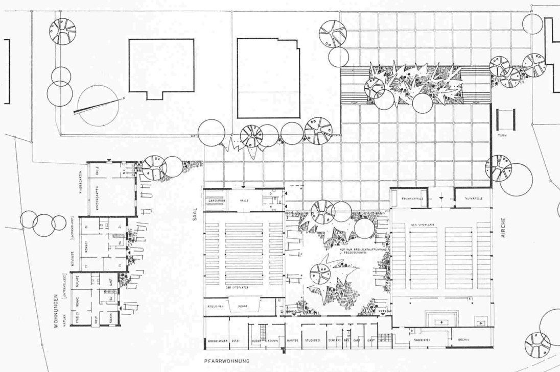
Erdgeschoss, Masstab 1:700
