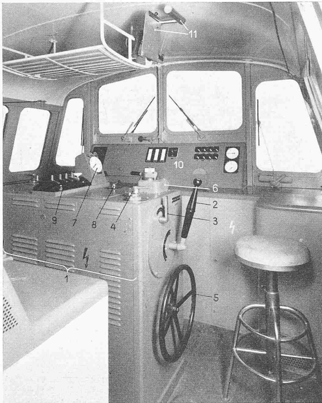
Bild 10. Führerstand der Bm 6/6-Lokomotive
