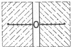
Bild 1. Ausgangsstellung (Einbauzustand)
