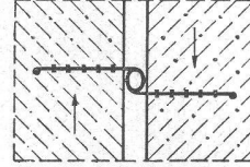
Bild 4. Scherbeanspruchung (Setzung)
