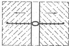
Bild 2. Zugbeanspruchung (Schwinden)
