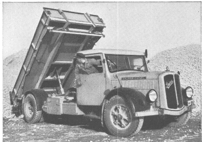
4 1-Dreiseitenkipper mit 4-Zylinder-Dieselmotor 29,6 Steuerpferde
