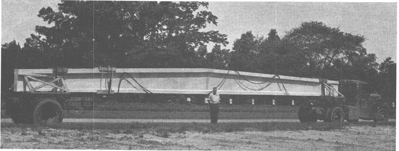
Vorfabrizierte, mit Spannkabeln BBRV vorgespannte Träger für Autohalle der Baum Chevrolet Co., Philadelphia
