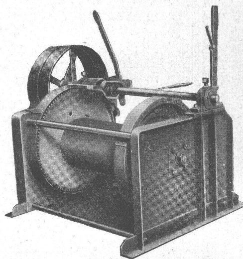
Seilwinde KS 23/70 mit gefrästem Stirnradgetriebe
