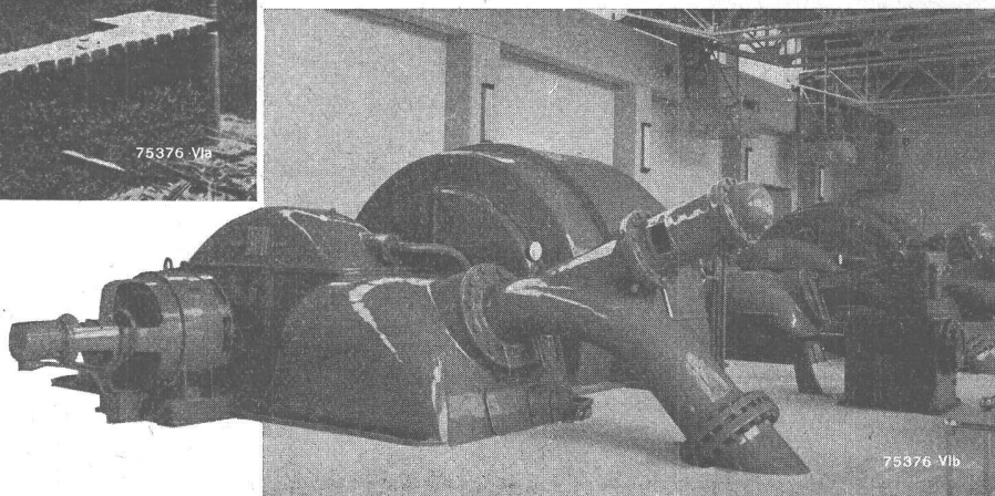
Aussenansicht und Maschinensaal des Wasserkraftwerkes «Juan Carlos», Moyopampa (Peru)
