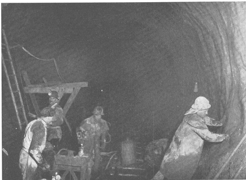
Abdichtungsarbeiten im Druckstollen von Verbano mit Sika 4a durch Arbeiter einer Unternehmung, die durch unsere Sika-Spezialisten angelernt wurden.
