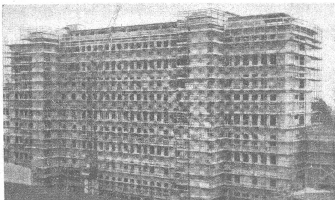
Bau- und Putzgerüst auf Konsolen 35 m hoch, Kantonsspital Zürich
